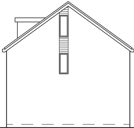
Dakkapel met platdak
